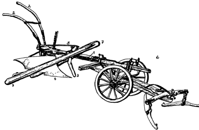
„Einflügler“ aus Natters Tir.: 1. Grindel, 2. Riester (Syn. → Störze), 3. Söck, 4. Wagense (Syn. → [Pflüg]schar), 5. Schnapper, 6. (Ge)rede, 7. Schleiße (nur für Ruhestellung und Transport des Pfluges).
