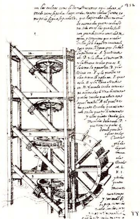
Dibuix de un «ingenio» para elevar el agua, que figura en la obra de Juanelo Turriano, Los veinte y un libros de los ingenios y máquinas (ca. 1564). Ms. 3372/3376 de la Biblioteca Nacional, Madrid.
